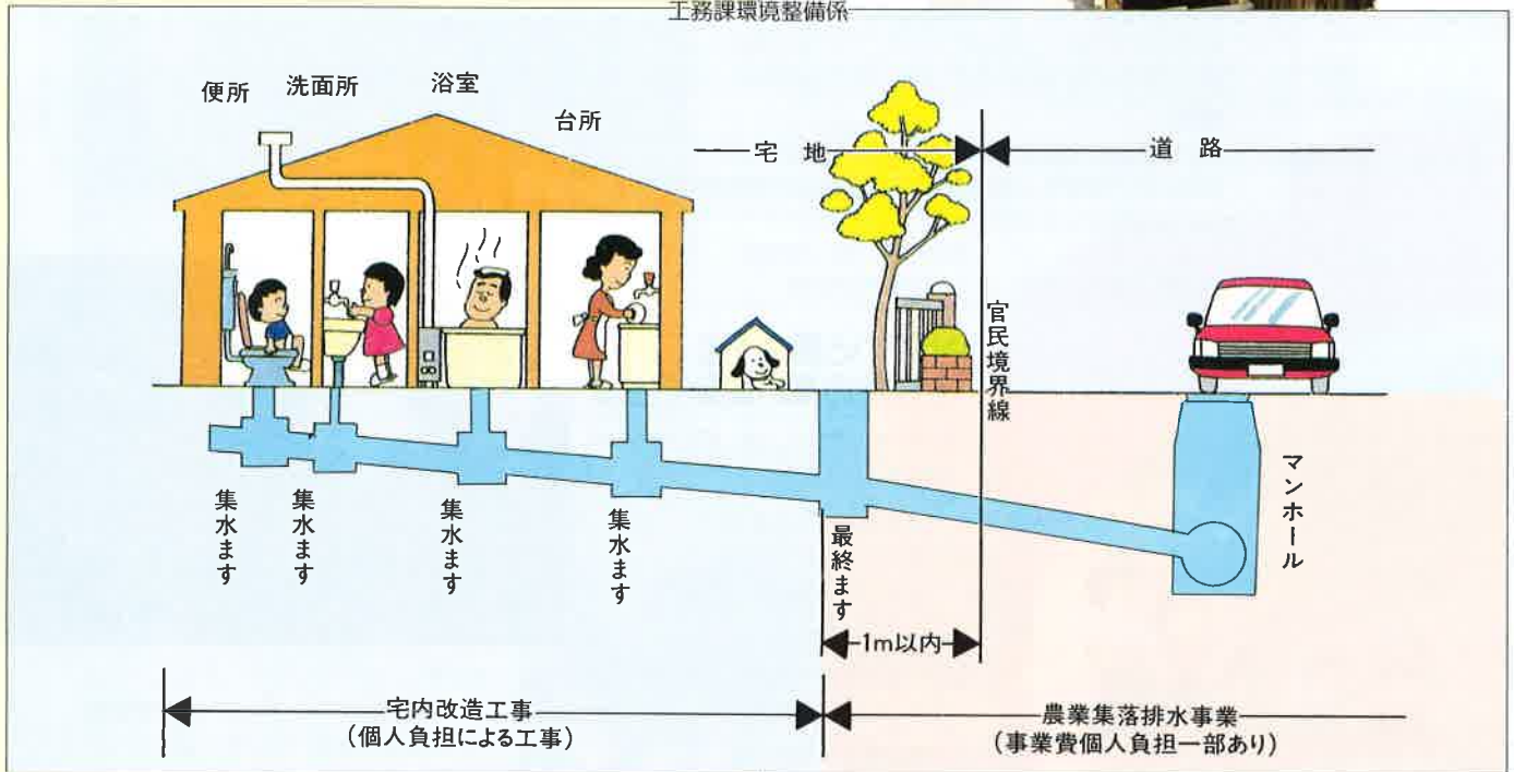
管路の工事
